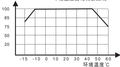
负载电流 (%) 环境温度变化减额曲线
